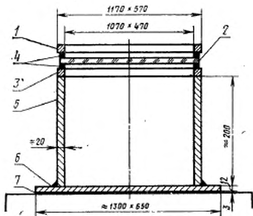
1 — верхняя рама; 2 — образец; 3 — нижняя рама; 4 — резиновые прокладки; 5 — коробка; 6 — стальной лист; 7 — армирующий лист
