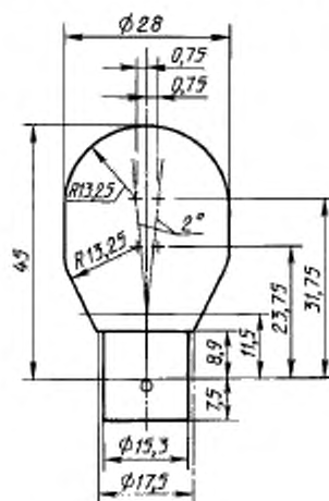
Черт. 4
