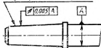
Конус Морзе по ГОСТ 9953-82
