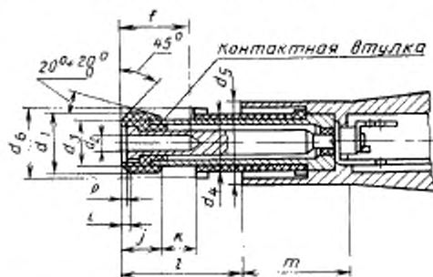
Размеры, мм
