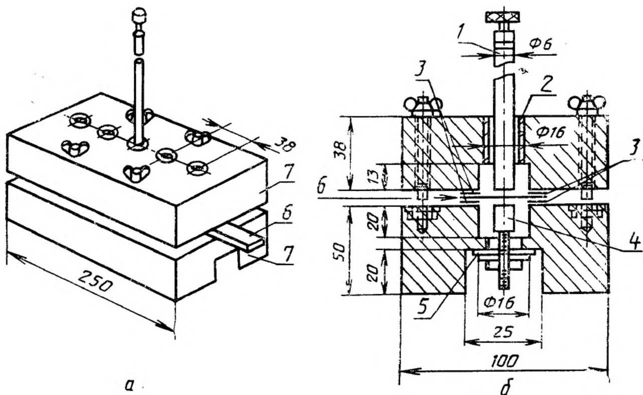
а — общая схема устройства; б — разрез устройства по электродам (верхняя часть слегка приподнята); 1 — верхний (подвижный) электрод; 2 — латунная втулка; 3 — лента из электр изоляционного материала; 4 — нижний электрод; 5 — латунная лента; 6 — образец; 7 — корпус из изоляционного материала
