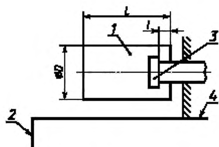
1 — соединитель; 2 — борт; 3 — приемно-отливной патрубков; 4 — палуба
