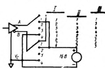
I — несправное состояние; II — переключение на провод А; III — установка на провод В
