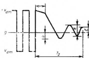
Общий вид периодических сигналов генератора
