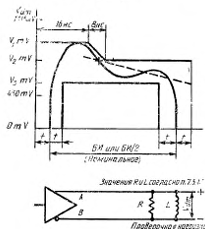
Дифференциальное выходное напряжение при нагрузке
