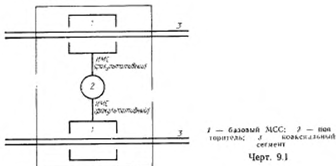
Повторительная установка, конфигурация коаксиал — коаксиал
