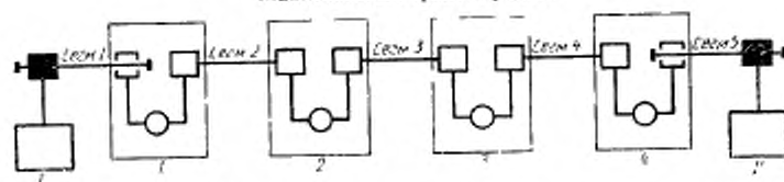
Максимальный тракт передачи
