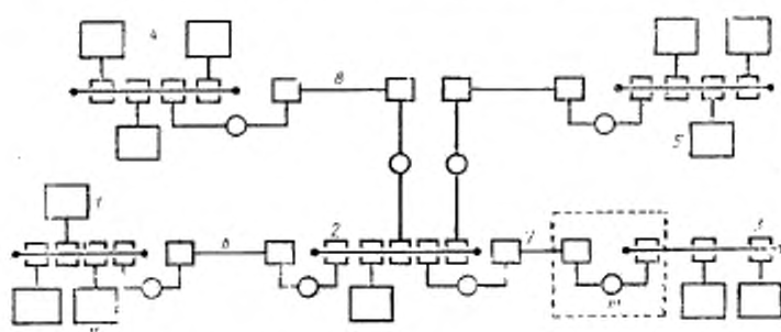
Пример большой системы с максимальными трактами передачи
