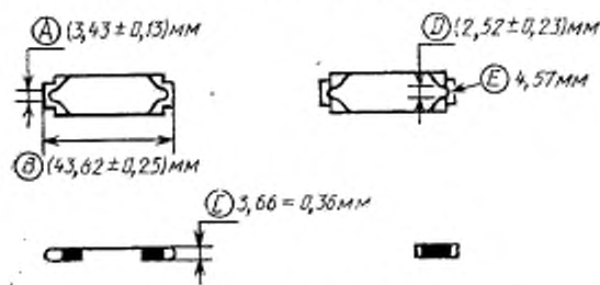
Скользящая защелка соединителя (максимальный размер материала 24)
