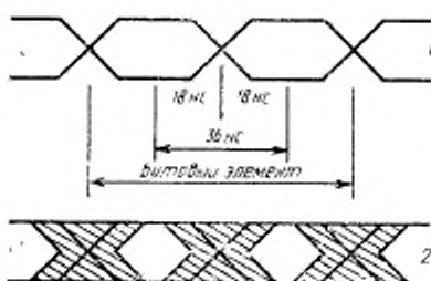
Изменение сигнала в наихудшем случае
