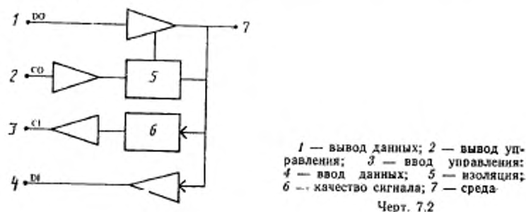
Общая модель МСС
