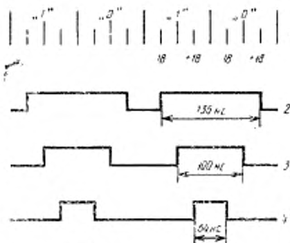
Изменение сигнала в наихудшем случае
