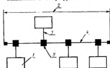
Минимальная конфигурация системы
