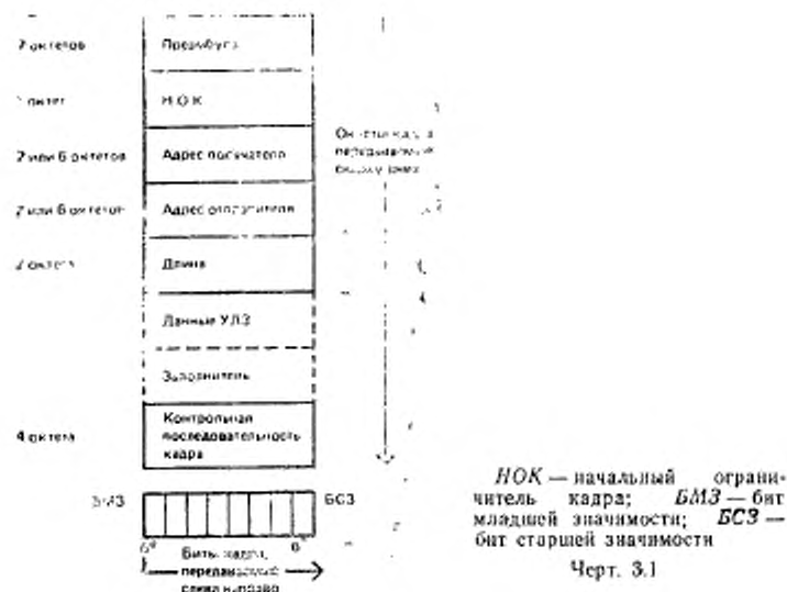
Формат кадра УДС
