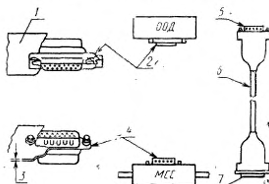
Детали соединителя и конфигурации кабеля ИМС
