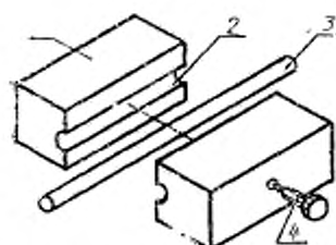
Общий вид коаксиального ответвительного соединителя
