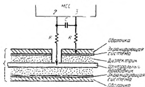
Типовая схема коаксиального ответвительного соединения
