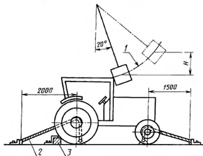
Пример крепления трактора. Удар спереди
