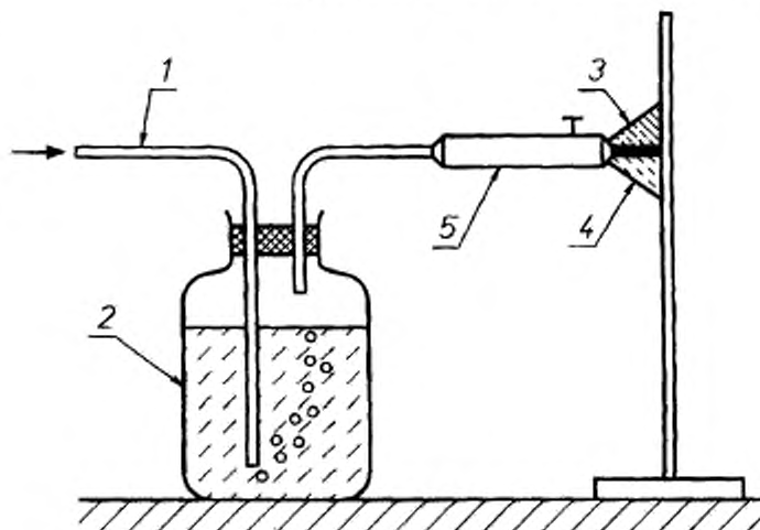
1 — трубка для подачи воздуха; 2 — бутылка; 3 — индикатор; 4 — форсунка газовой смеси; 5 — ручка с АКТИВНЫМ ЭЛЕКТРОДОМ
