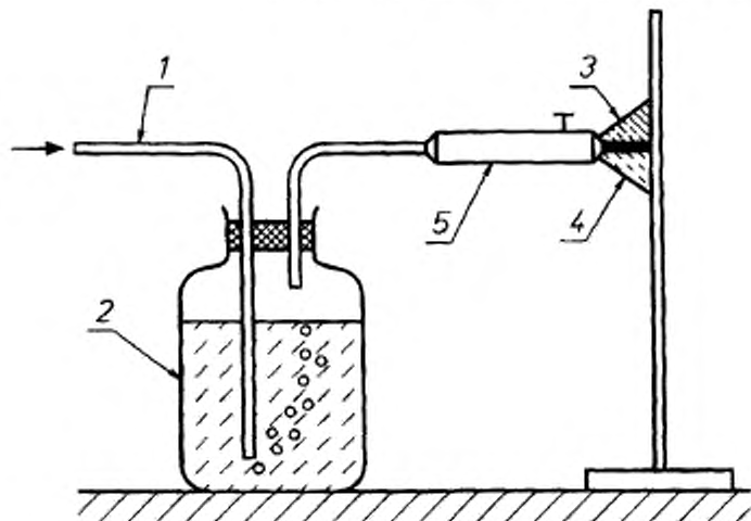
1 — трубка для подачи воздуха; 2 — бутылка; 3 — индикатор; 4 — нозонка газовой смеси; 5 — ручка с АКТИВНЫМ ЭЛЕКТРОДОМ
