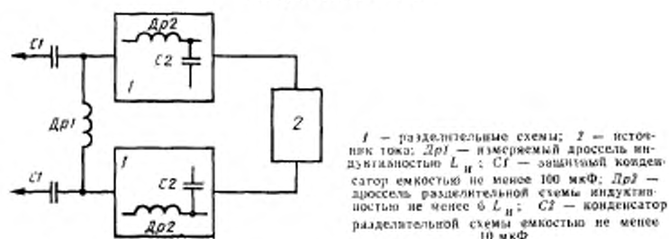
Измерительная схема
