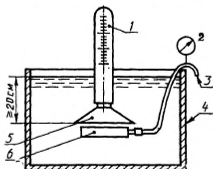
1—градуированный цилиндрический сосуд (п. 8.2.3); 2—манометр для измерения испытательного давления; 3—газопровод; 4—водяная ванна (п. 8.2.1); 5— воронка (п. 8.2.4); 6—испытательное устройство
