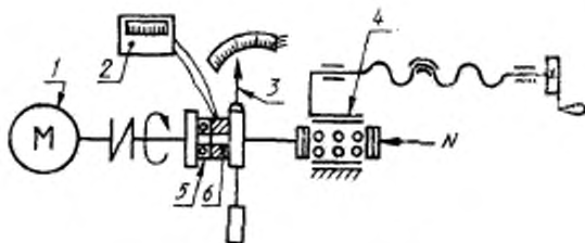
1 — двигатель; 2 — потенциометр; 3 — маятниковый склони- метр; 4 — нагружающее устройство; 5 — фрикционный образец; 6 — металлический образец
