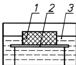
1 — образец; 2 — сетчатая подставка; 3 — ванна с водой
