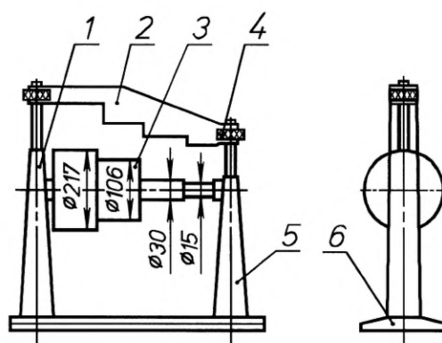
1 — опора; 2 — прижимная планка; 3 — цилиндр; 4 — гайка; 5 — опора; 6 — основание
