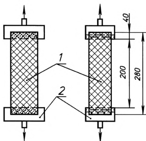
1 — образец; 2 — игольчатый зажим
