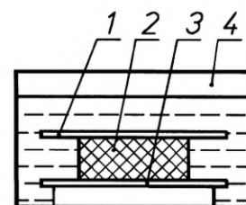
1 — сетчатый пригруз; 2 — образец; 3 — сетчатая подставка; 4 — ванна
