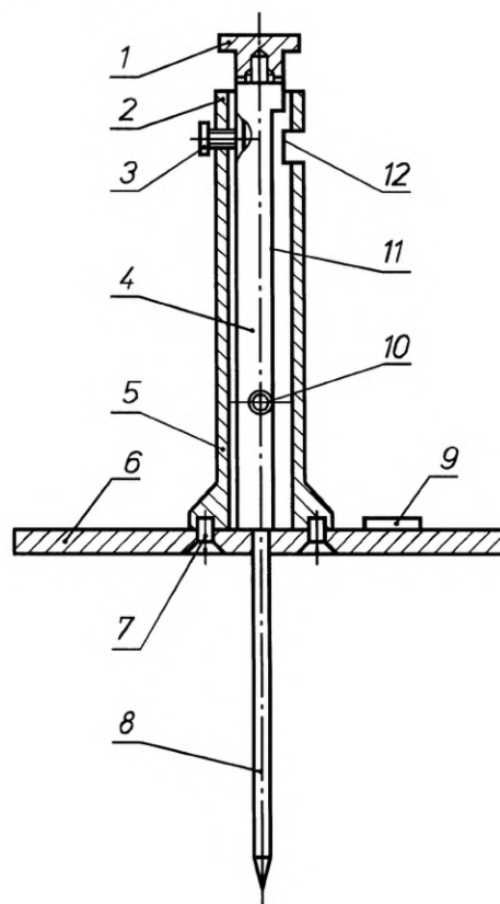
1 — ручка; 2 — втулка; 3 — зажимной винт; 4 — вставка; 5 — корпус; 6 — основание; 7 — крепежный винт; 8 — игла; 9 — табличка; 10 — крепежный винт; 11 — шкала; 12 — стекло
