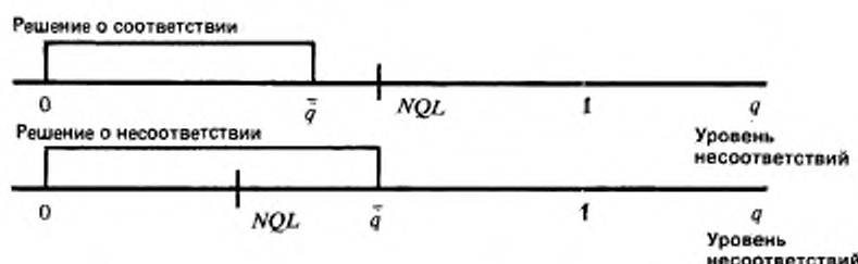
Рисунок 1 — Правила принятия решений при контроле поставщика по методу доверительных границ
