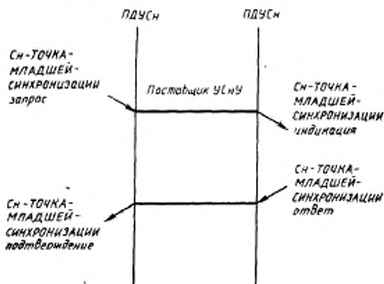
Рисунок 13 — Последовательность примитивов услуги Сн-ТОЧКА-МЛАДШЕЙ-СИНХРОНИЗАЦИИ
