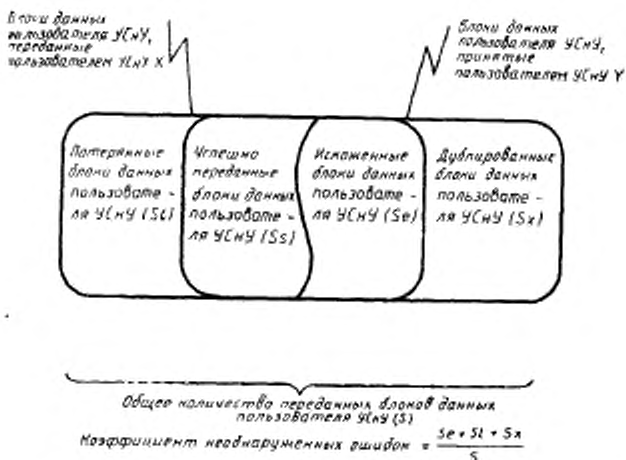
Рисунок 4 — Компоненты коэффициента необнаруженных ошибок
