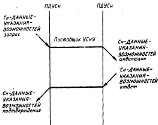
Рисунок 9 — Последовательность примитивов услуги Сл-ДАННЫЕ-УКАЗАНИЯ-ВОЗМОЖНОСТЕЙ
