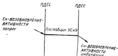
Рисунок 19 — Последовательность примитивов услуги ВОЗБНОВЛЕНИЕ-АКТИВНОСТИ
