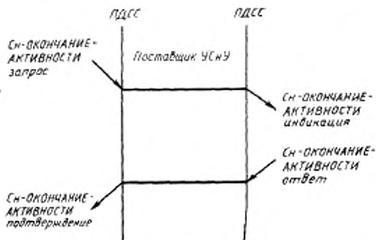
Рисунок 22 — Последовательность примитивов услуги СН-ОКОНЧАНИЕ-АКТИВНОСТИ
