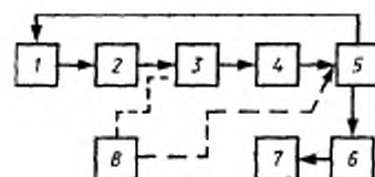
1 — анализатор боковых полос по 6.2.2; 2 — передатчик; 3 — согласованная нагрузка по 6.2.3; 4 — аттенуатор дополнительный; 5 — согласованный тройник; 6 — демодулятор по 6.2.1; 7 — осциллограф по 6.2.6; 8 — направленный ответвитель по 6.2.4
