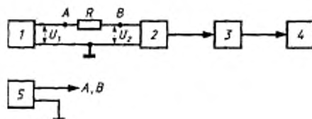
1 — генератор сигналов НЧ по 6.2.8; 2 — передатчик; 3 — элемент затенения по 6.2.3; 4 — девиометр по 6.2.9; 5 — вольтметр НЧ по 6.2.10; R — измерительное сопротивление 600 Ом \pm 0,5\%
