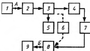
1 — генератор ТВ измерительных сигналов по 6.2.5; 2 — переключатель; 3 — тройниковый переход для подключения ВЧ головки вольтметра; 4 — эквивалент антенны с фиксированным аттенуатором по 6.2.3; 5 — ВЧ вольтметр по 6.2.11; 6 — направленный ответитель по 6.2.4; 7 — дополнительный аттенуатор; 8 — демодулятор по 6.2.1; 9 — осциллограф по 6.2.6
