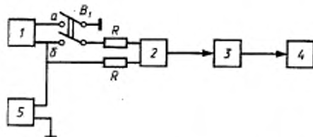
1 — генератор сигналов НЧ по 6.2.8; 2 — передатчик; 3 — эквивалент антенны по 6.2.3; 4 — девиометр по 6.2.9; 5 — вольтметр НЧ по 6.2.10; R — измерительное сопротивление 300 Ом \pm 0,2 \%
