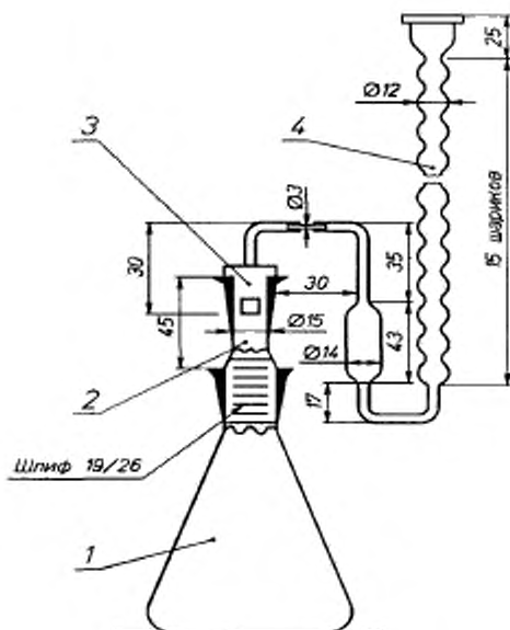
1 – коническая колба вместимостью 100 см³; 2 – насадка для positioning электрода; 3 – резиновая пробка; 4 – абсорбер для поглощения АШН, изготовленный по указанным размерам.
