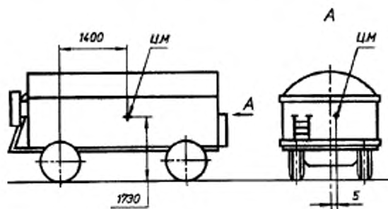
Рисунок 1 — Центр массы электростанции
