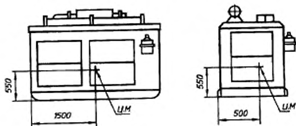
Рисунок 2 — Центр массы электроагрегата
