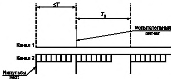
Рисунок 6 — Измерение длительности задержки ( T_1 ) у ЭКС R-синхронизированного типа
