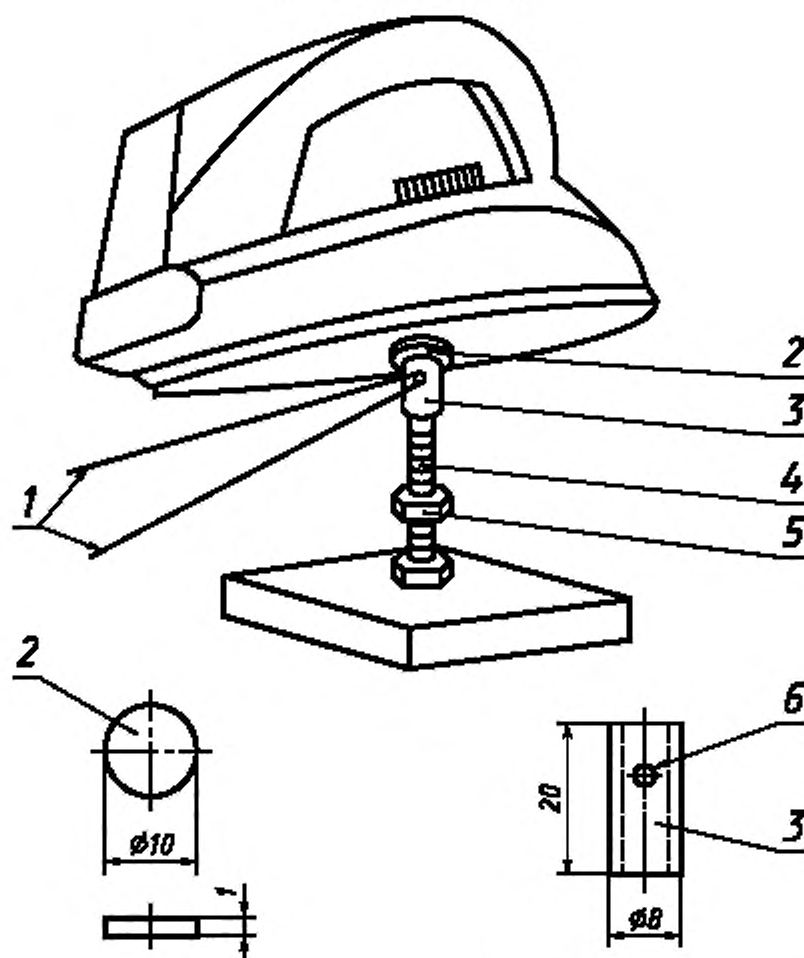
1 — выводы термонары; 2 — диск термонары; 3 — керамическая втулка; 4 — пружина; 5 — регулировочная гайка; 6 — отверстие для присоединительных проводов термонары
