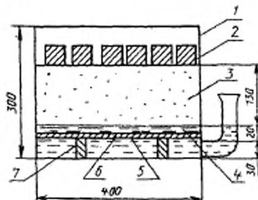
1 — сосуд; 2 — образцы; 3 — капиллярно-увлажненный песок; 4 — вода; 5 — фильтровая бумага; 6 — металлическая сетка; 7 — подставка
