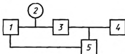
1 — генератор модулированных скачков сигнала (В.1.2.15); 2 — вольтметр (В.1.2.1.3); 3 — УЗЧ; 4 — эквивалент нагрузки (В.1.2.8); 5 — осциллограф (В.1.2.16)
