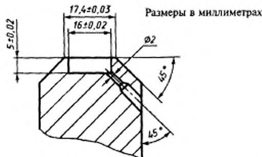
Рисунок 2 — Устройство из закаленной стали для приготовления образцов для испытания (требуется две такие детали)
