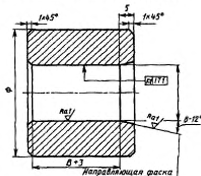
Рисунок 7 — Кольцевой калибр
