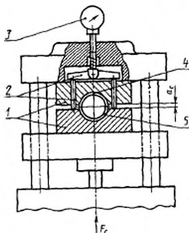
1 — контрольный блок; 2 — система передачи величины измерения; 3 — измерительный прибор с круговой шкалой; 4 — разъем; 5 — втулка
