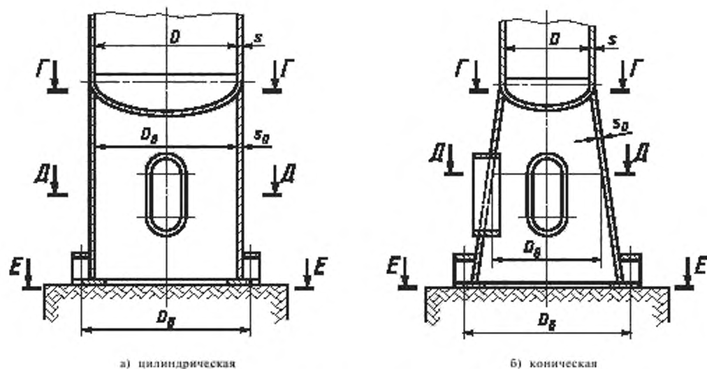
Рисунок 2 — Расчетные сечения опорной обечайки
