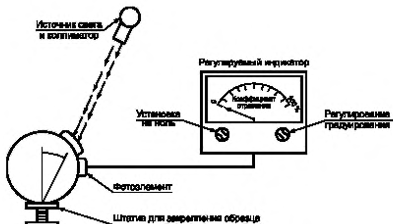
Рисунок 4.2 — Общая схема оборудования для измерения отражающей способности с использованием в приемном устройстве шара Ульриха
