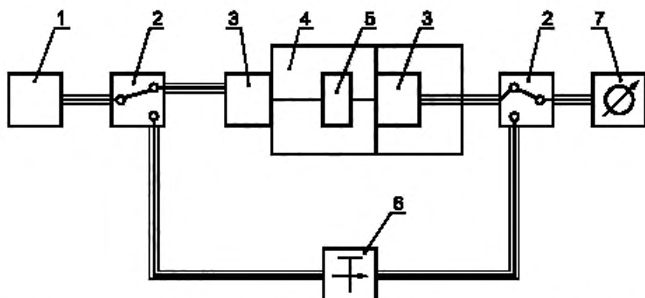
1 — генератор сигналов; 2 — коаксиальный переключатель; 3 — фиксированный Т-аттенуатор (10 дБ); 4 — испытательный контейнер; 5 — испытуемый образец; 6 — откалиброванный регулируемый аттенуатор; 7 — измерительный прибор
