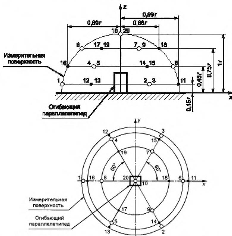
Рисунок Б.2 — Точки измерения на полусферической измерительной поверхности
