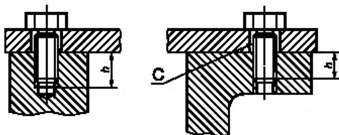
Рисунок 1 — Допуски и зазор для резьбовых крепежных деталей
