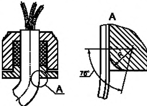
Рисунок В.2 — Скрутка кромок в месте ввода гибкого кабеля
