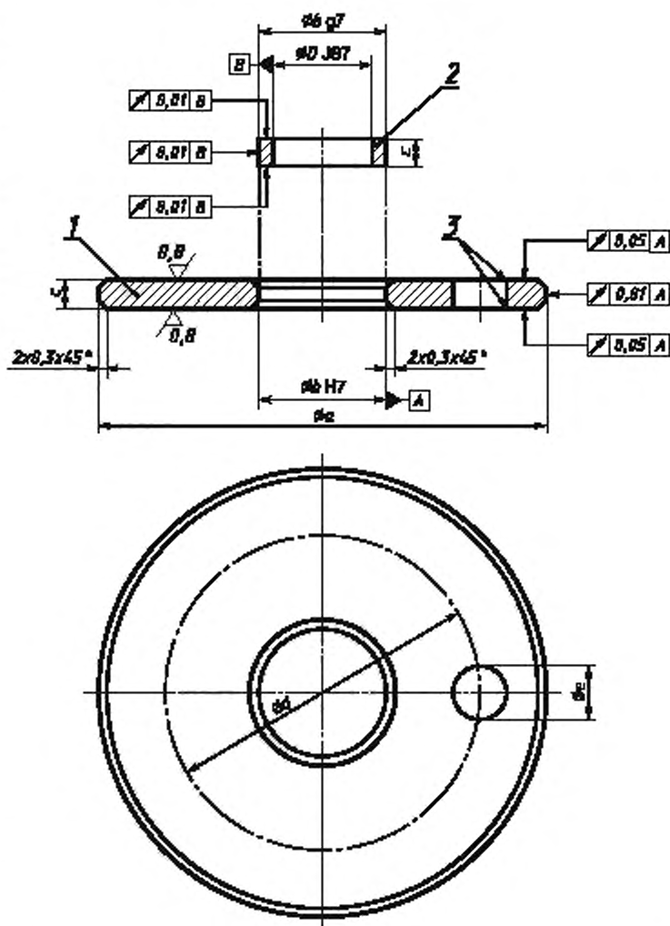
Рисунок 4 — Конструкция имитатора испытательного крута и промежуточной втулки
