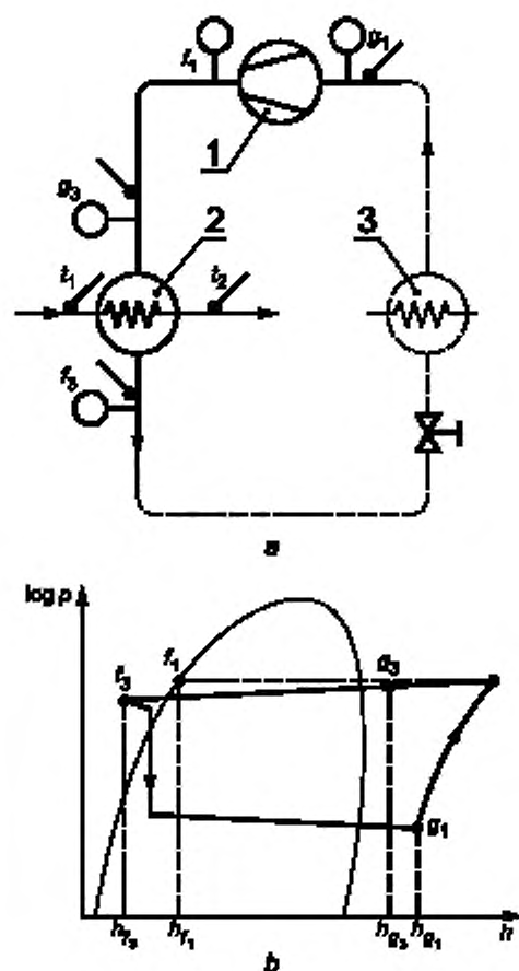
а — схема цикла; б — диаграмма \log p-h
