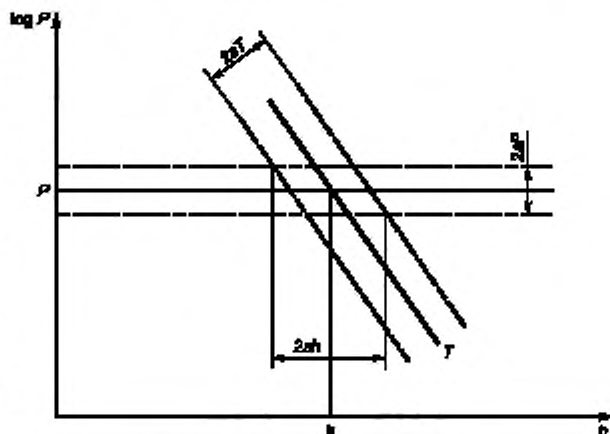
Рисунок В1 — Диаграмма \log p-h
