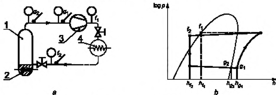
a — схема цикла; б — диаграмма \log p-h
