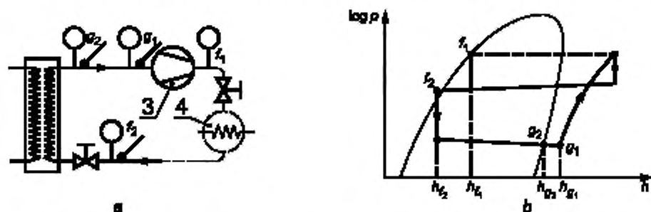
a — схема цикла; б — диаграмма \log p-h
