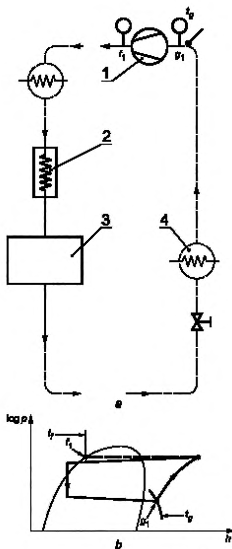
а — схема цикла; б — диаграмма \log p-h
