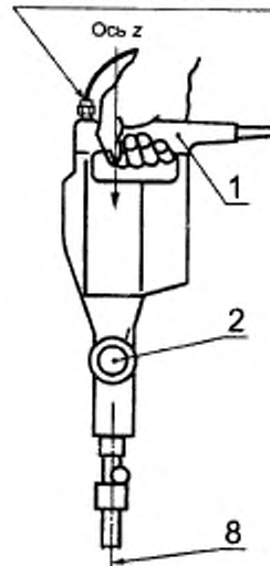
Рисунок 1 — Направление измерений; положение и крепление датчика
