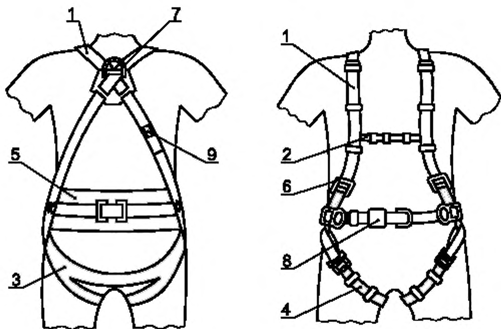
1 — наплечная лямка; 2 — вспомогательная лямка; 3 — задняя лямка (основная); 4 — набедренная лямка; 5 — задняя опора для регулирования рабочего положения; 6 — регулирующий элемент; 7 — элемент крепления; 8 — пряжка; 9 — маркировка
