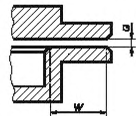
Рисунок 2 — Плоское соединение
