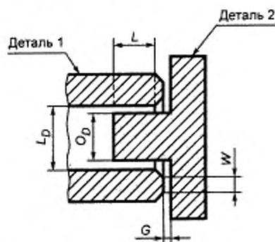
Рисунок 3 — Цилиндрическое соединение
