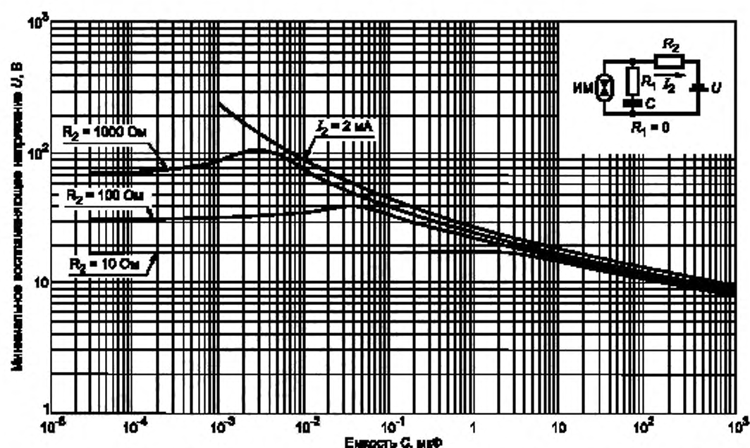
Рисунок А.12 — Минимальное воспламеняющее напряжение в активизированной взрывоопасной водородно-кислородной смеси (81 % H_2 + 19 % O_2 ) для емкостных цепей подгруппы IIА при R_1 = 0 Ом
