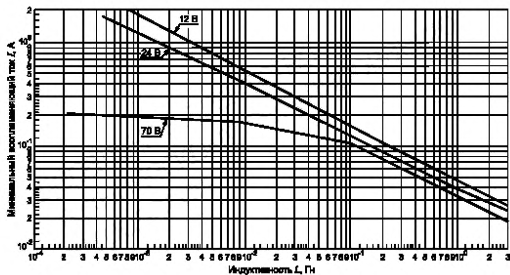
Рисунок А.7 — Индуктивные цепи группы I
