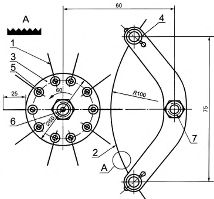
Рисунок Б.9 — Кинематическая схема искрообразующего механизма II типа
