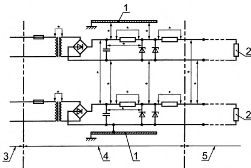
1 — шасси; 2 — нагрузка; 3 — искробезопасная цепь, заданная U_n ; 4 — часть искробезопасной цепи, не являющаяся искробезопасной; 5 — искробезопасная цепь; * — расстояния разделения, в отношении которых применяется таблица 4
