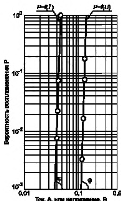
Рисунок А1.5 — Зависимости вероятности воспламенения от значения воспламеняющего тока или напряжения. Электрические схемы контрольных цепей
