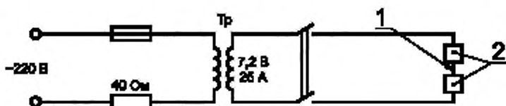
Рисунок Б.8 — Принципиальная электрическая схема устройства подготовки вольфрамовых проволок методом оплавления
