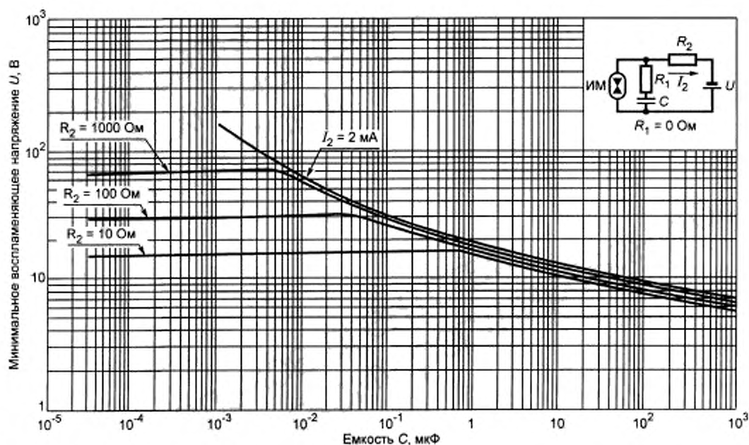
Рисунок А.16 — Минимальное воспламеняющее напряжение в активизированной взрывоопасной водородно-кислородной смеси (75 % H_2 + 25 % O_2 ) для емкостных цепей подгруппы ПВ при R_1 = 0 \text{ Ohm}
