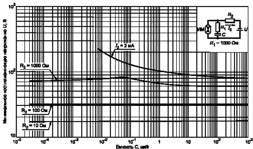
Рисунок А.15 — Минимальное воспламеняющее напряжение в активизированной взрывоопасной водородно-кислородной смеси (81 % H_2 + 19 % O_2 ) для емкостных цепей подгруппы ПА при R_1 = 1000 \text{ Ohm}
