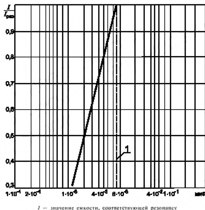
Рисунок А1.16— Зависимость снижения воспламеняющего тока ( I ) относительно воспламеняющего тока при резонансе ( I_{рас} ) от емкости при постоянных индуктивностях и частотах
