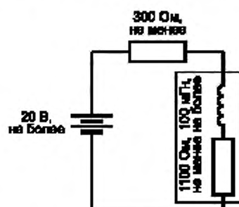
Рисунок А.23 — Простая индуктивная цепь
