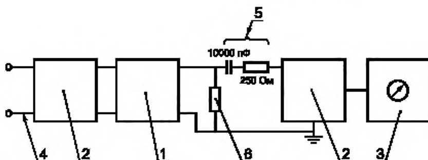
1 — устройство питания электрического заграждения; 2 — V-образный эквивалент сети (см. 5.1.2); 3 — измеритель ИРП; 4 — провода к сети электропитания или к батарее; 5 — элементы эквивалентной схемы ограждения (полное сопротивление нагрузки обеспечивается резистором сопротивлением 250 Ом, соединенным последовательно с сопротивлением 50 Ом V-образного эквивалента сети); 6 — резистор утечки сопротивлением 500 Ом (следует добавить в эквивалентную схему 5)
