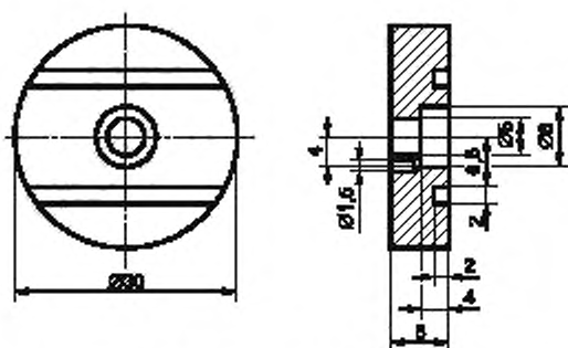
Рисунок 3 — Кадмиевый контактный диск
