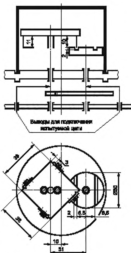
Рисунок 2 — Кинематическая схема искробразующего механизма I типа
