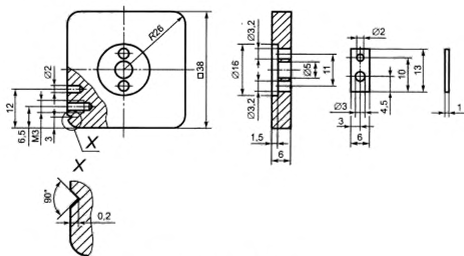
Рисунок 4 — Держатель проволоки
