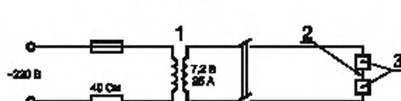
1 — трансформатор с площадью поперечного сечения сердечника 19 см 2 ; 2 — вольфрамовая проволока; 3 — медные бруски
