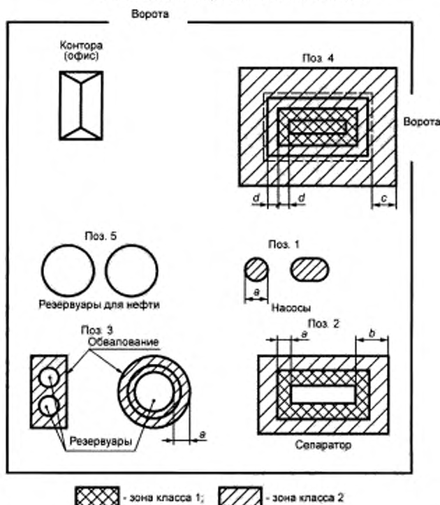
Пример № 11 Резервуарный парк для бензина и нефти
