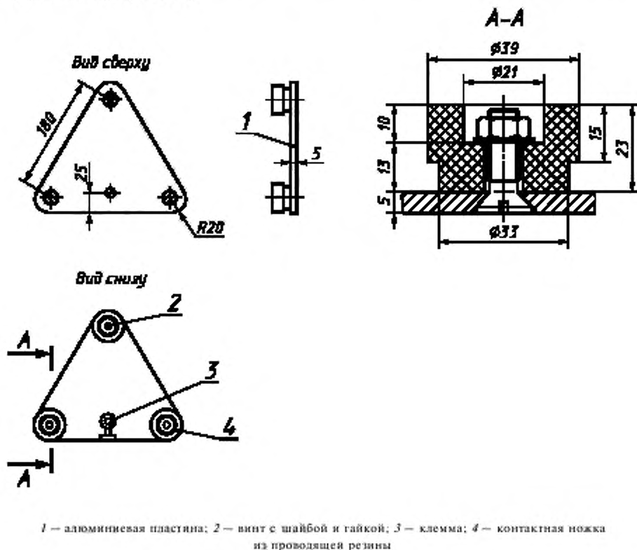
Рисунок А.1 — Испытательный электрод 2
