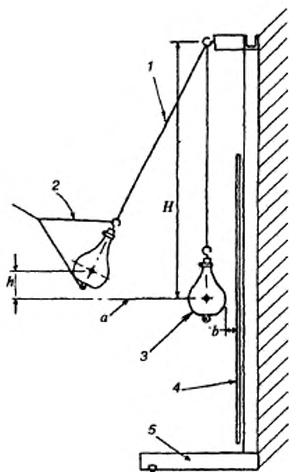
1 — стальной трос диаметром 2,5 — 4 мм; 2 — узелка для подъема мешка; 3 — кожаный мешок (мягкое тело); 4 — испытываемый образец, закрепленный в стенде; 5 — опора; H — высота подвеса; h — высота падения мешка; a — центральная ось испытываемого образца; b — расстояние между образцом и мешком, висящим в свободном состоянии
