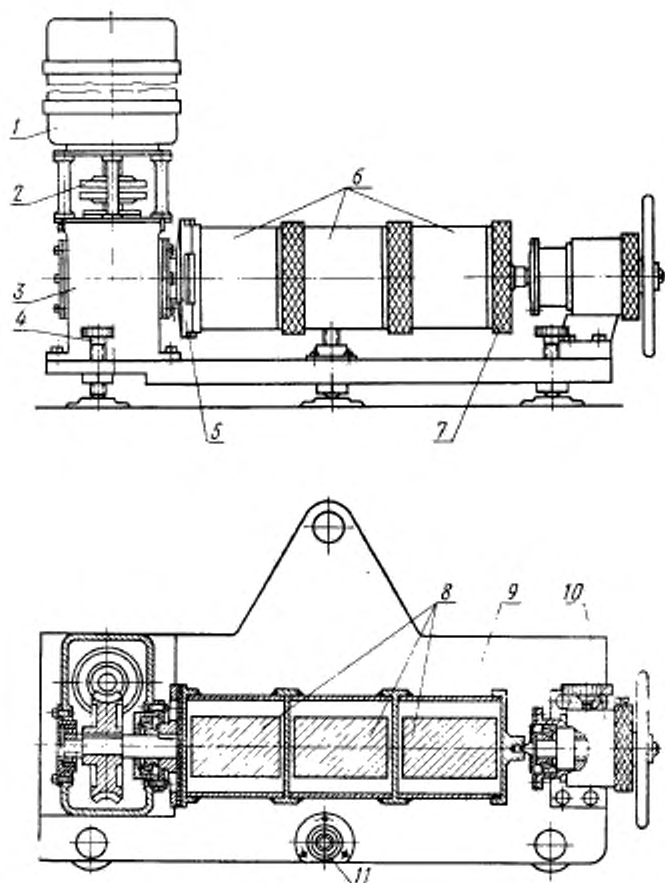
1—электродвигатель; 2—муфта; 3—червячный редуктор; 4—регулирующий винт; 5—плиты; 6—барабаны; 7—крышка; 8—истирающие стержни; 9—плита; 10— задняя бабка; 11—уровень.
