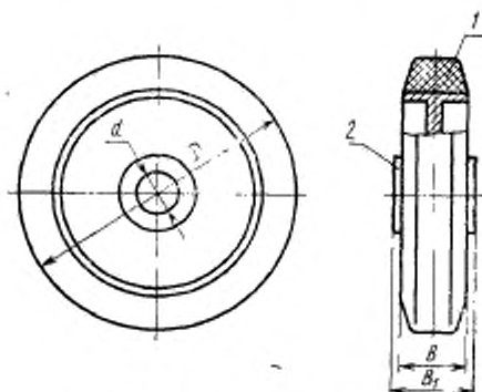
1—шина по ГОСТ 5883—78; 2—обод-ступица.
