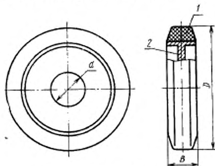
1—шина по ГОСТ 5883-76; 2—обод.
