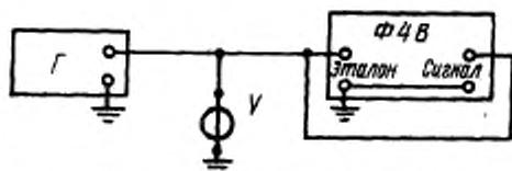
Г—измерительный генератор; V—образцовый вольтметр; Ф4В—поверяемый фазочувствительный вольтметр.
