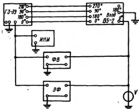
Схема поверки вольтметра В5—2
