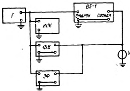
Схема поверки вольтметра В5—1
