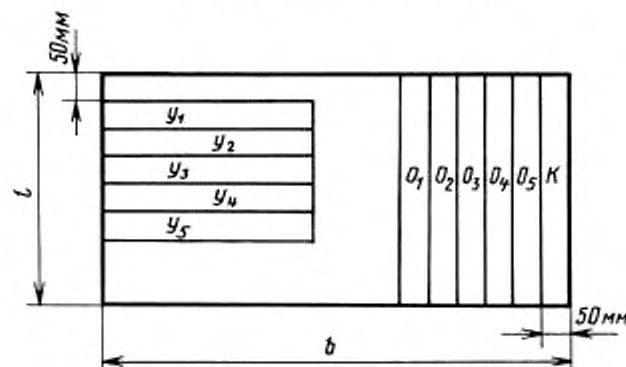
Схема раскроя элементарных проб
