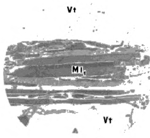
Сросток микролитотипа 1-й группы ( V_t ) + + каолинит ( Ml_1 ) Черт. 7
