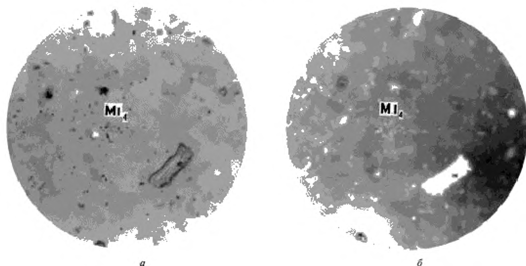
Известняк (МІ 4 ) (увеличение 200)
