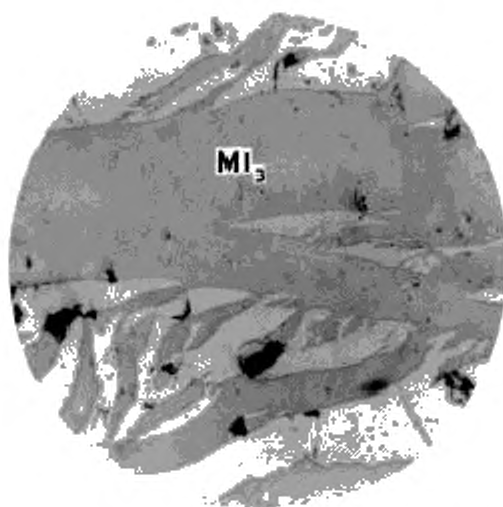
Сидерит по трещинам ( MI_3 ) (увеличение 200)
