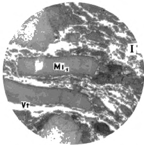
Сросток микролитотипа 2-й группы ( V_t + P ) + + каолинит ( MI_1 )
