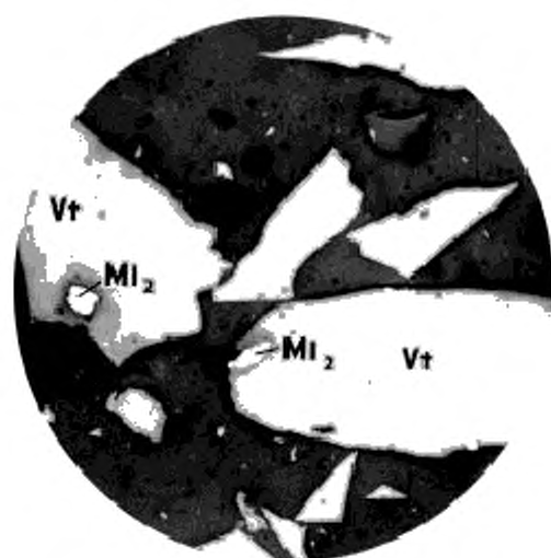
Сростки микролитотипов 1-й группы (V) + + пирит (Ml 2 )
