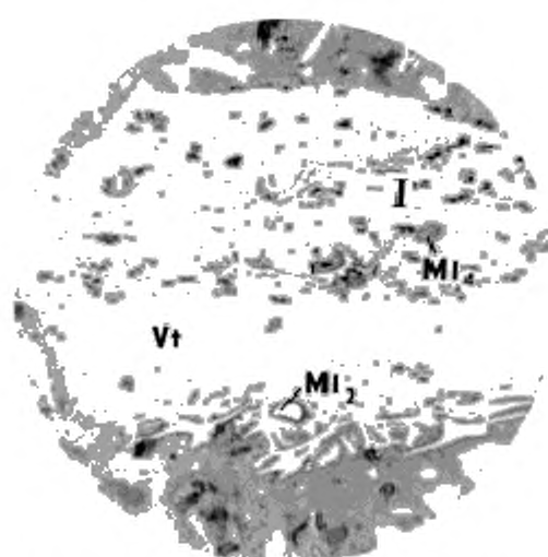
Сросток микролитотипа 2-й группы (V + F) + + кварц (Ml 1 ) + пирит (Ml 2 )
