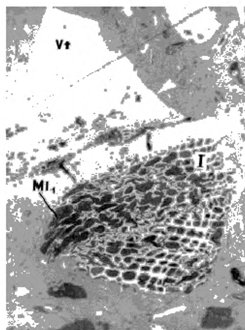
Сросток микролитотипа 2-й группы ( V_t + P ) + аргиллит ( Ml_1 ) Черт. 6
