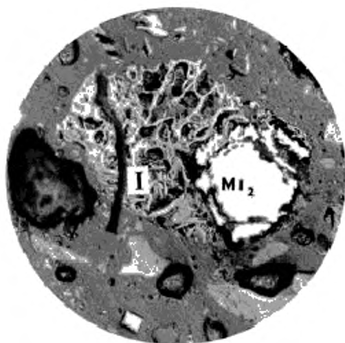
Сросток микролитотипа 3-й группы ( P ) + + пирит ( MI_2 )
