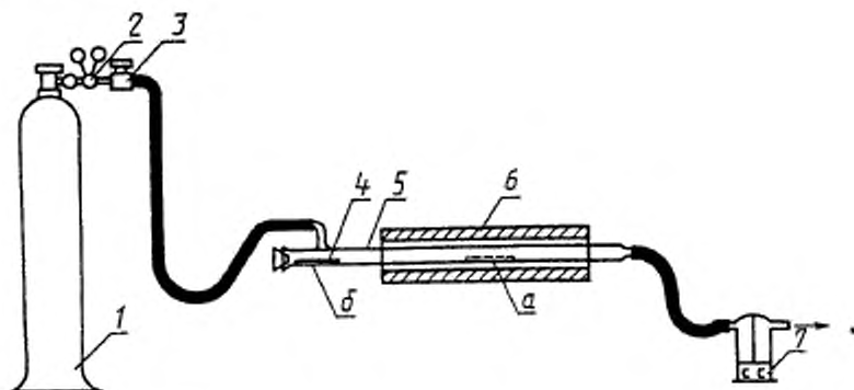
1 — баллон с инертным газом; 2 — редуктор; 3 — вентиль тонкой регулировки; 4 — лодочка фарфоровая для пробы; 5 — трубка кварцевая; 6 — печь электрическая трубчатая; 7 — склянка Типенко с дистиллированной водой
