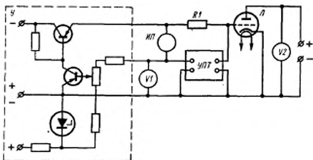
Y — одна из возможных схем транзисторного стабилизатора напряжения; V1, V2 — вольтметры постоянного тока; ИП — измерительный прибор; УПТ — усилитель постоянного тока; R1 — резистор; Л — испытываемая лампа.
