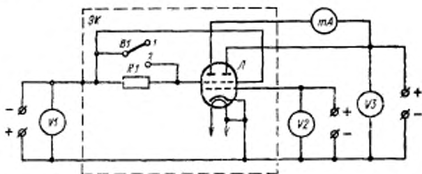
V1 , V2 , V3 —вольтметры постоянного тока; mA —миллиамперметр постоянного тока; B1 —выключатель; R1 —резистор; Л —испытываемая лампа; ЭК —экранирующая камера.
