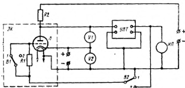
V1, V2 —вольтметры постоянного тока; ИП —измерительный прибор; R1, R2 —резисторы; B1 —выключатель; B2 —переключатель; УПТ —усилитель постоянного тока; L —испытуемая лампа; ЭК —экранирующая камера.
