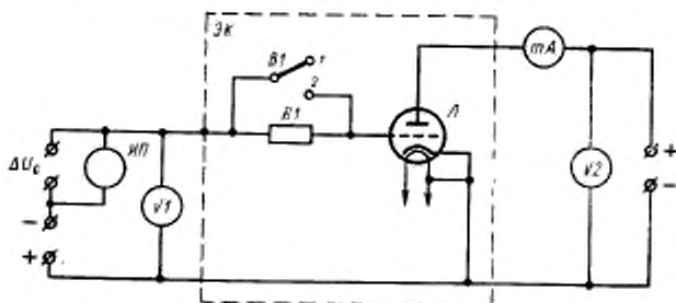
V1 , V2 —вольтметры постоянного тока; mA —миллиамперметр постоянного тока; ИП —измерительный прибор; B1 —выключатель; R1 —резистор; Л —испытываемая лампа; ЭК —экранирующая камера.
