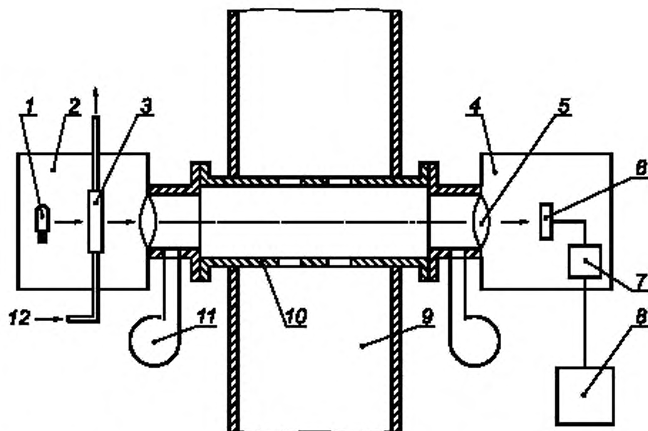
1 — источник излучения; 2 — излучатель; 3 — внутренняя калибровочная ячейка; 4 — приемник; 5 — защитное окно; 6 — детектор; 7 — электронный модуль; 8 — блок регистрации данных; 9 — газопровод или труба; 10 — труба для настройки или калибровки; 11 — нагнетатель продувочного воздуха; 12 — трубка для подачи калибровочного газа
