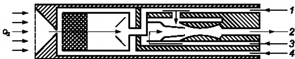
1 — область пониженного давления зонда; Q_2 — расход разбавляемого газа/пробы ( Q_2 ); 2 — расход разбавленной пробы ( Q_1 + Q_2 ); 3 — расход газа-разбавителя/воздуха ( Q_1 ); 4 — продувка калибровочным газом/воздухом
