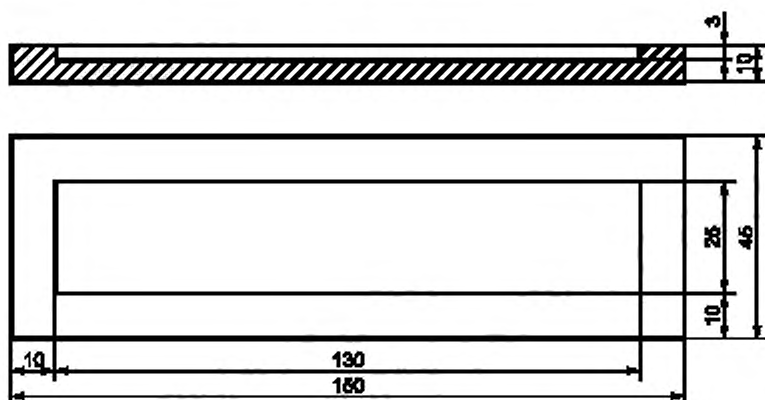
Рисунок 3 — Лоток для определения рабочего времени оттискового материала
