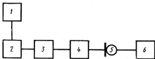
1—частотомер; 2—генератор; 3—магазин затухания; 4—электростатический возбудитель; 5—поверный микрофон; 6—электронный вольтметр.
